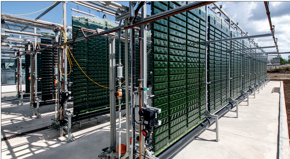
180-Liter-Reaktormodule der Freilandanlage am Fraunhofer CBP in Leuna (© Fraunhofer IGB). | Bild in Farbe und Druckqualität: www.fraunhofer.de/presse .
