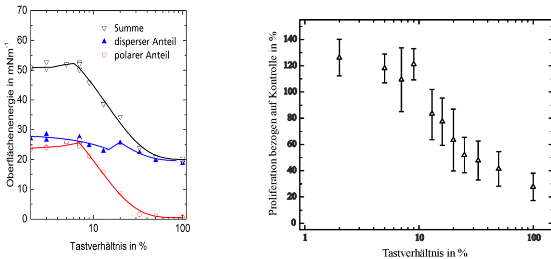
Abbildung 2: links: Oberflächenspannung in Abhängigkeit vom Tastverhältnis des Beschichtungsverfahrens. Das Tastverhältnis bestimmt hier den Bedeckungsgrad mit einer Beschichtung niedriger Oberflächenspannung rechts: Besiedelung der nach linkem Abbildungsteil hergestellten Oberfläche mit primären Fibroblasten nach drei Tagen[1,2].
