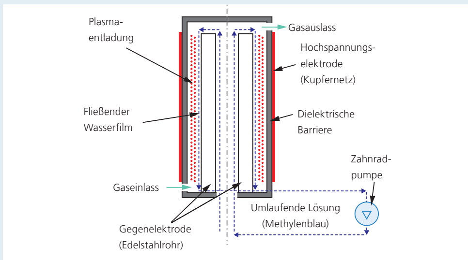
Schematischer Aufbau eines Plasmareaktors zur Wasserbehandlung.
